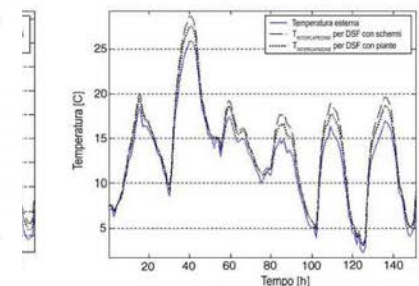
Fig. 9 - Valori della temperatura dell'aria e della parete interna per la facciata a doppia pelle con gli schermi e con le piante. (Fonte: W.G. Stec, A.H.C., Van Paassen, A. Maziarz. Grafico rielaborato dall'autore.)
