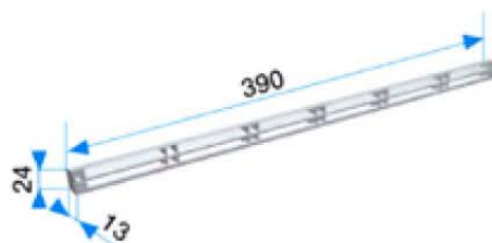
Controvento standard
